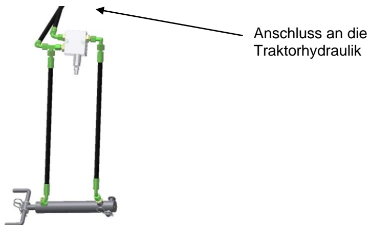
Bild 15 Anschluss der hydr. Strommengenregulierung
